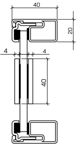
CROISILLONS COLLÉS 40mm LOFT20
