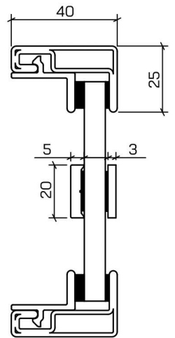
CROISILLONS COLLÉS 20mm LOFT 25
