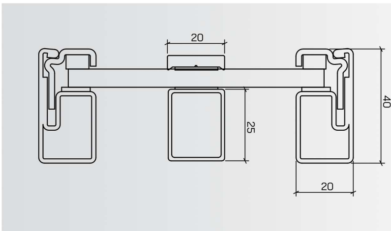
CROISILLONS COLLÉS 20mm LOFT 35
