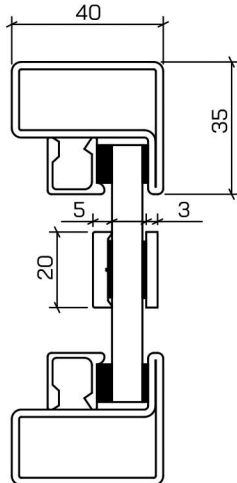
CROISILLONS COLLÉS 20mm LOFT 35
