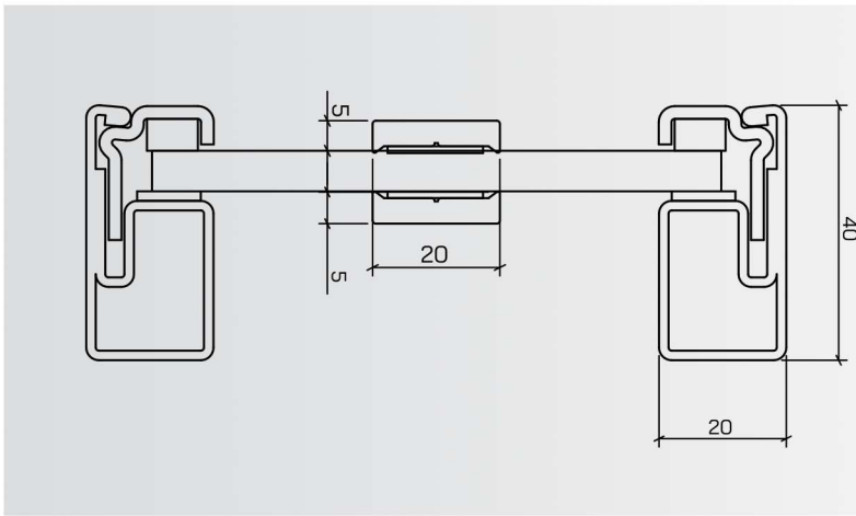
CROISILLON SOUDÉ D'UN CÔTÉ 20mm | LOFT 20
